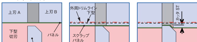
①トリムライン切断開始 ②トリムライン切断完了 ③スクラップカットライン切断完了
